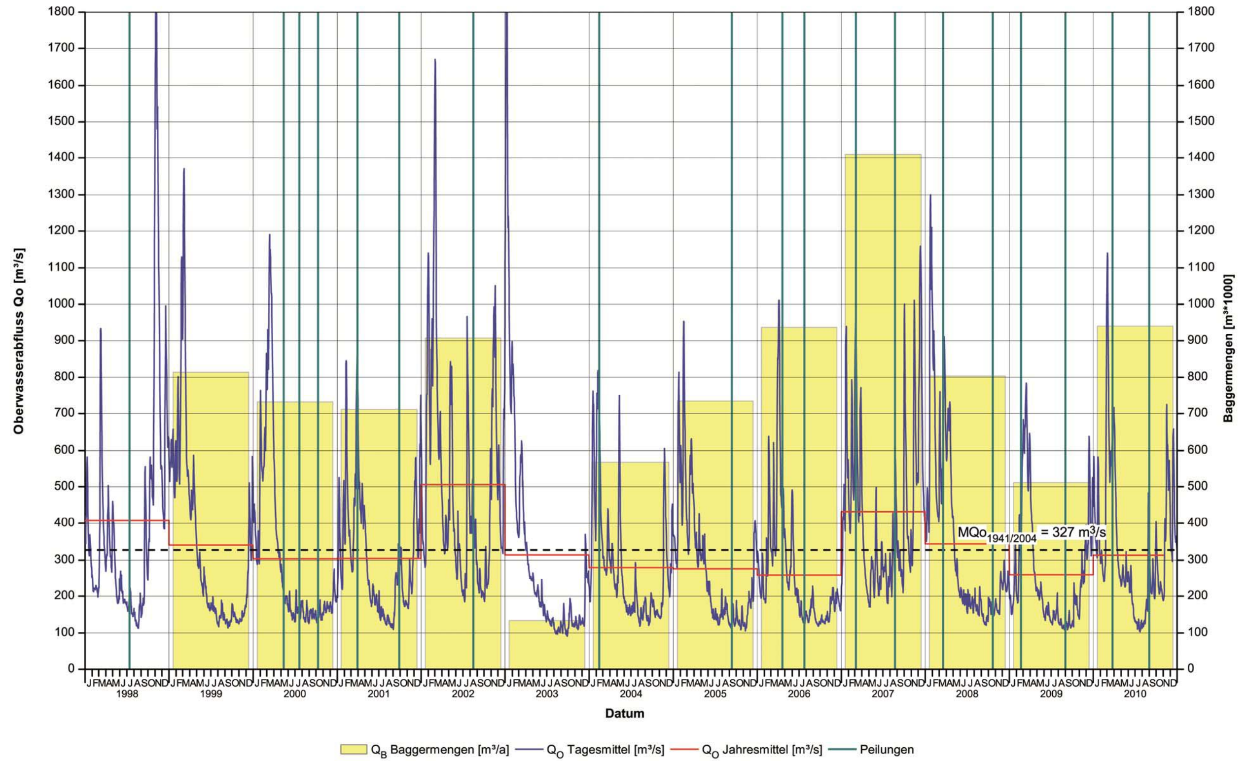
Abb. 2: Oberwasser am Pegel Intschede [20], Baggerungen [21] und Fahrrinnenpeilungen [1] bis [19] 1998 bis 2010
